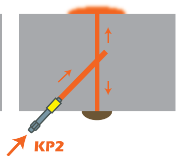
④注入： 市販のグリスポンプで注入をします。 クラックが充填されると目止めの脇 から樹脂が漏出します
